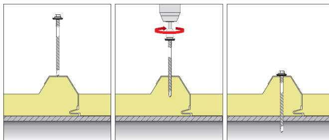
Montáž střešního sendvičového panelu na povrch (při volbě délky šroubu zohledněte výšku horní plochy panelu, který má být upevněn)
